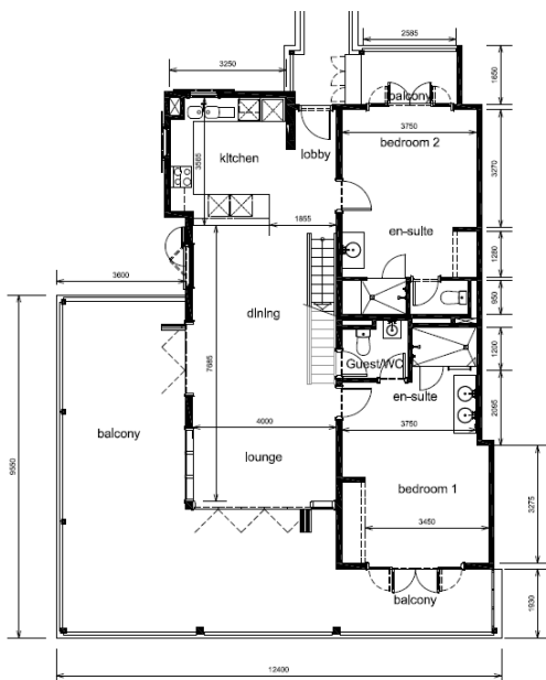
Půdorys hlavního patra:
