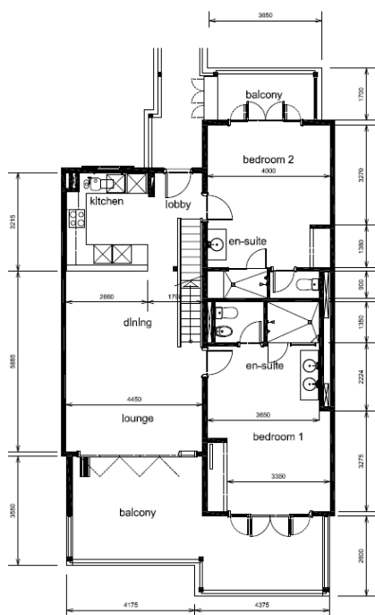
Půdorys spodního patra:
