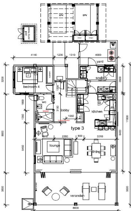
Půdorys přízemí:
