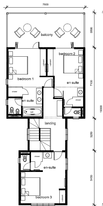
Půdorys 1. patra
