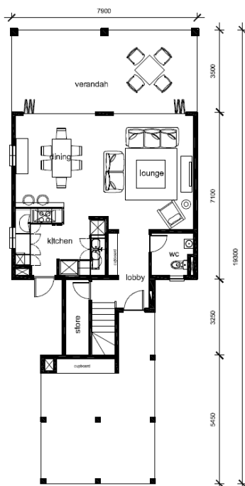
Půdorys přízemí
