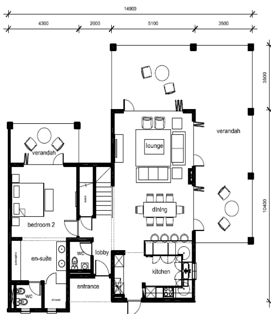
Půdorys přízemí:
