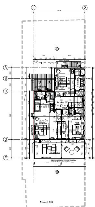
Půdorys 1. patra:
