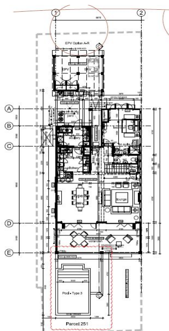
Půdorys přízemí:
