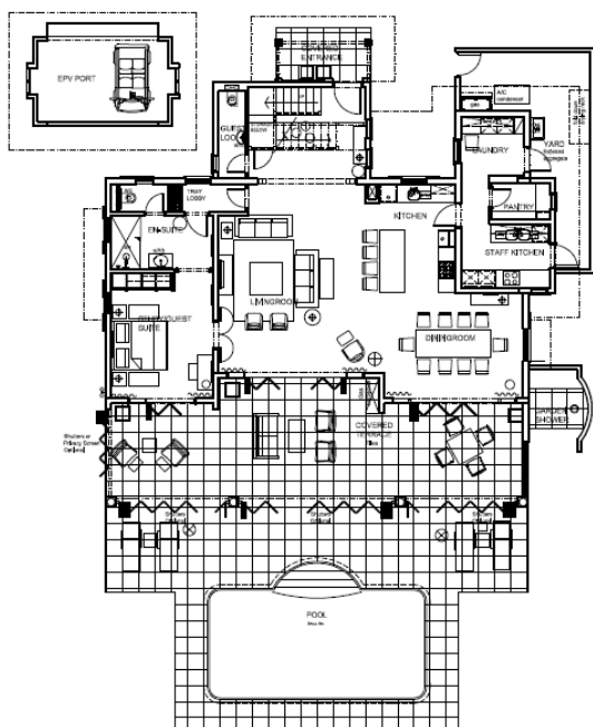
Půdorys přízemí:
