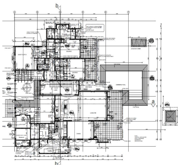
Půdorys přízemí
