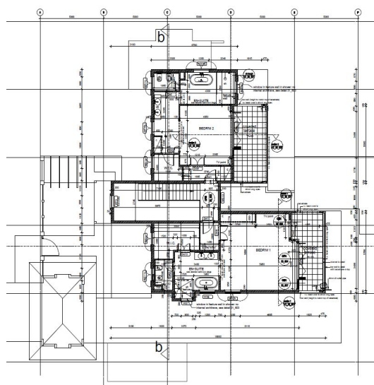
Půdorys 1. patra
